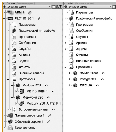
Рис. 1. Дерево физической структуры проекта с подключаемым оборудованием в MasterSCADA 4D
