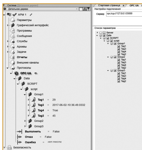
Рис. 3. Редактор OPC UA в MasterSCADA 4D
